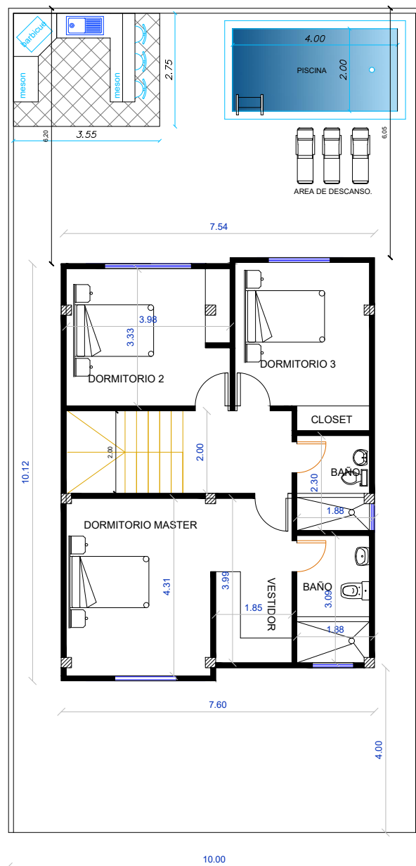
VILLA ARENA 2 PLANTA NIVEL +3.00
