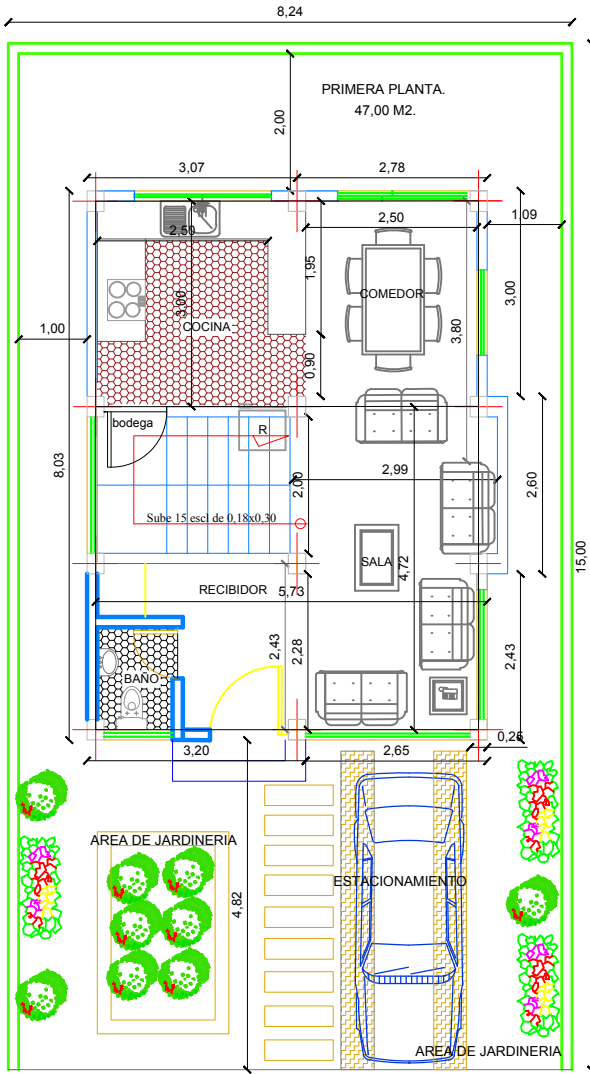
PLANTA BAJA N+0.30
