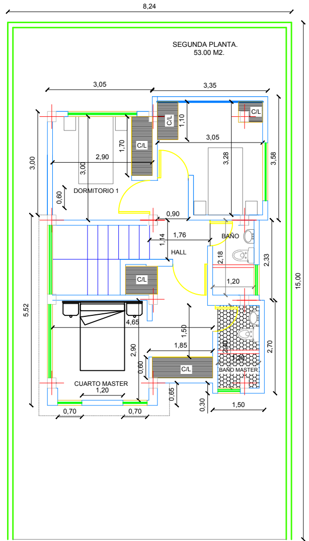
PLANTA NIVEL +3.00
